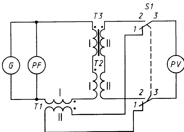
Рисунок 1 — Схема для измерений в динамическом режиме перемангничивания
